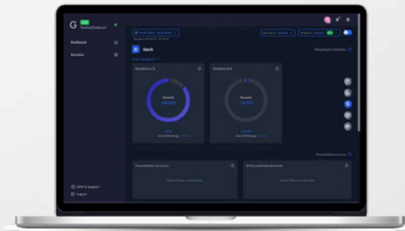
KPIs
